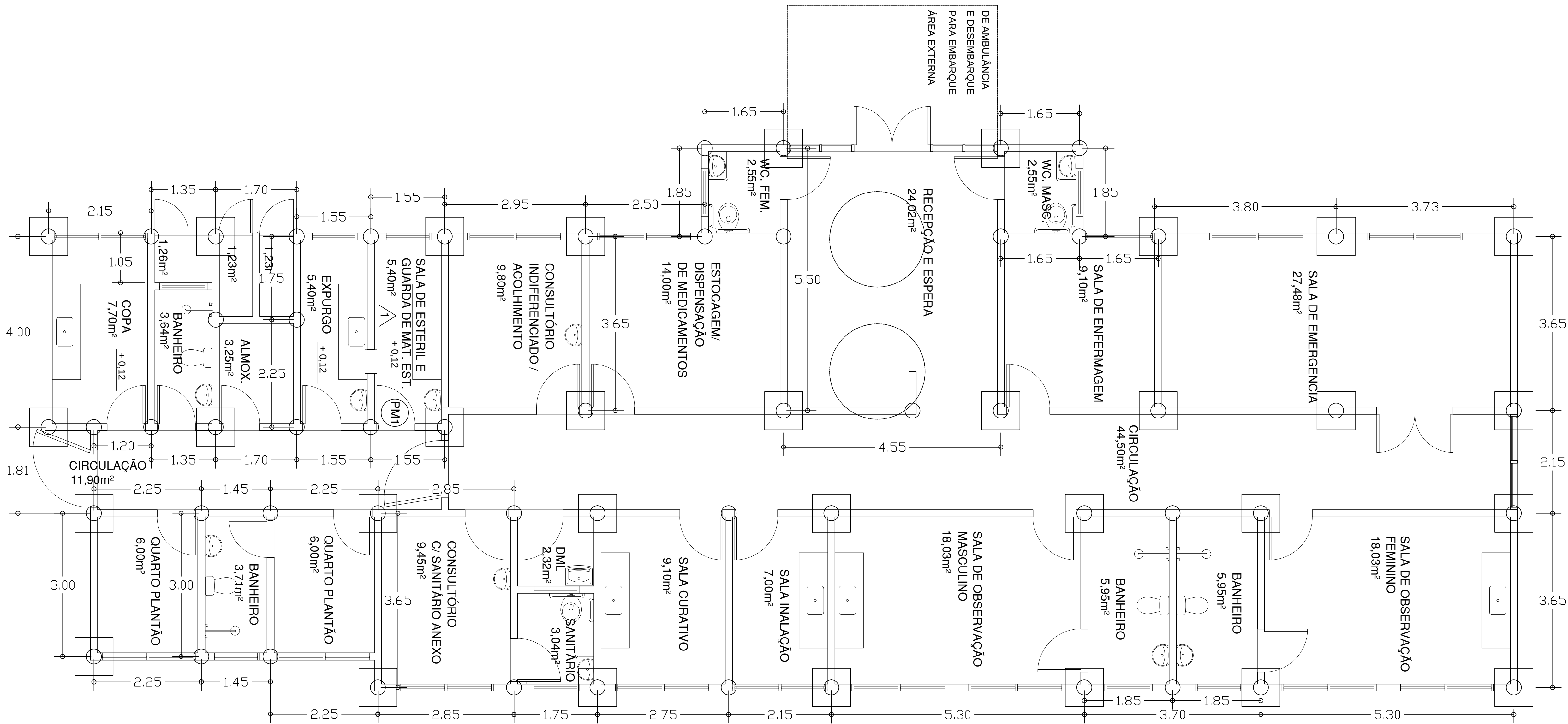
PLANTA DE ESTRUTURA Esc. 1:50
